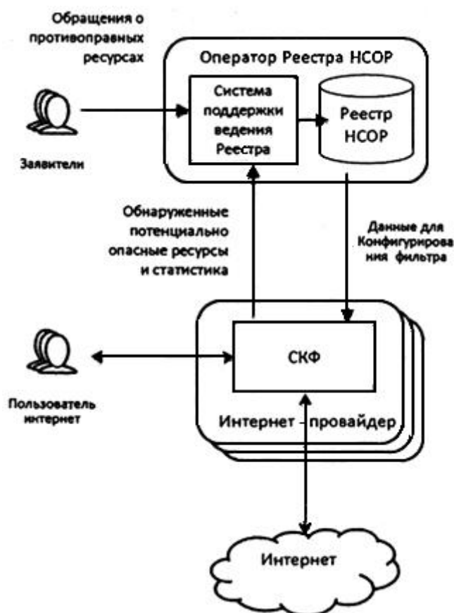
Рис. 6. Принцип контроля доступа через Реестр НСОР
