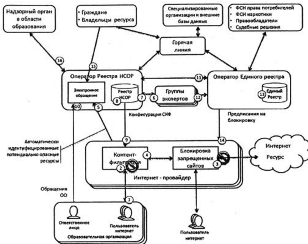
Рис.1. Схема процесса взаимодействия
