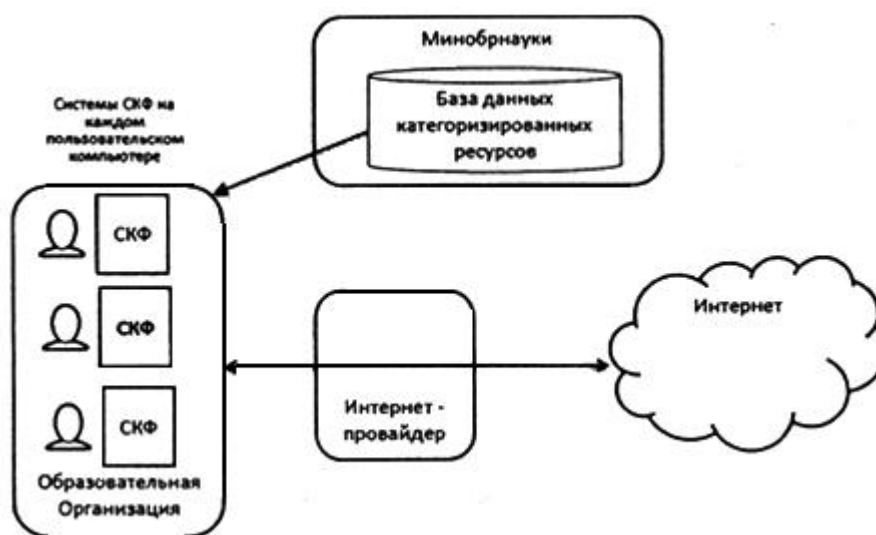
Рис.3. Схема работы контент-фильтрации при размещении в ОО
